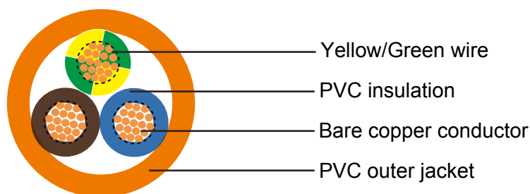
H03V2V2-F
